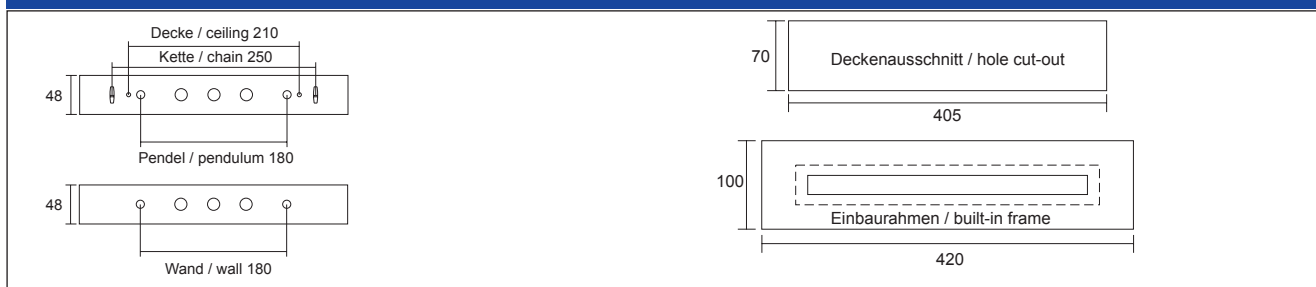
Bohrabstände KX Wand / Decke Drilling distances KX wall / ceiling
